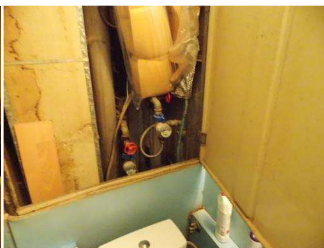
inštalačné jadro s meračmi vo WC
